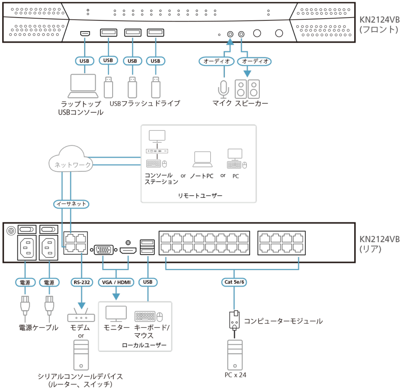
構成図
